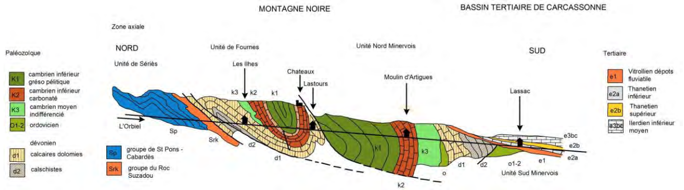
Fig 2 : Coupe synthétique schématique du Minervois E.Monceret 2007, d'après G.M Berger et al. Feuille de Carcassonne 1993.
