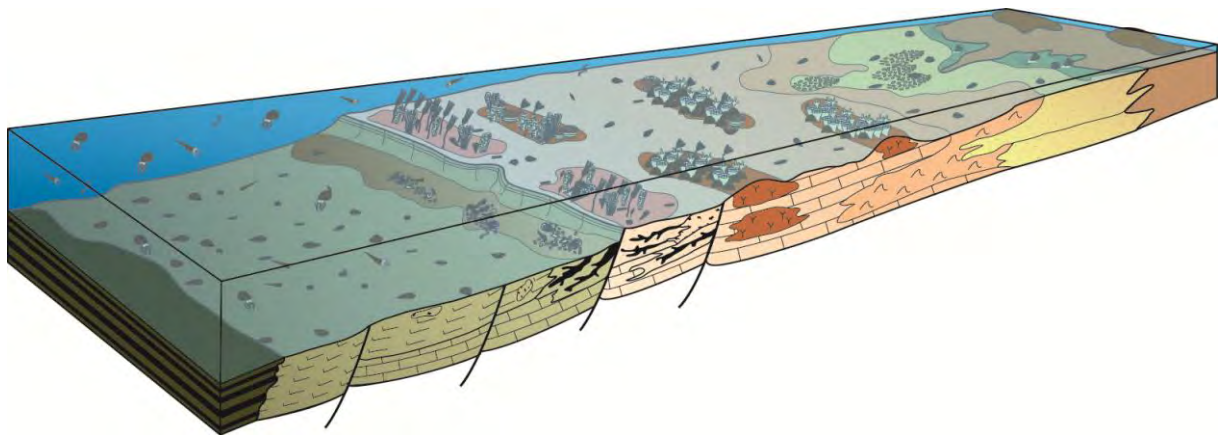
Fig 3 : Paléoenvironnement du Dévonien des marbrrières de Caunes Minervoises d'après M.Dilax et al. 2016
