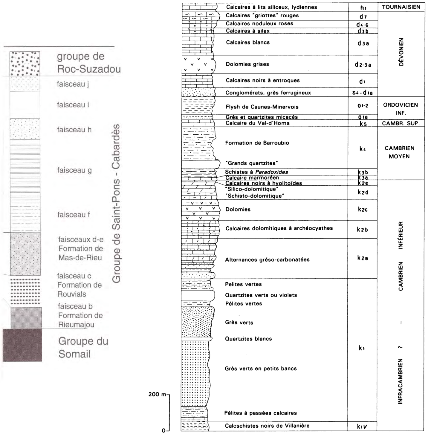
Fig. 2 - Colonne stratigraphique synthétique de la série paléozoïque de la nappe du Minervois
