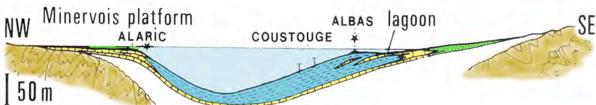
Esquisse paléogéographique de la bordure nord-pyrénéenne au Paléocène.
