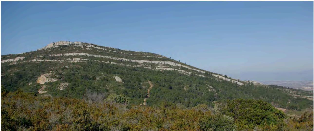
Versant nord de l'anticlinal de l'Alaric au Sud de Moux.
