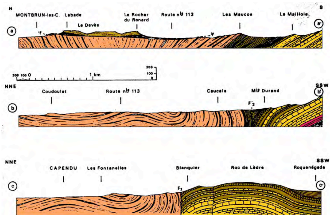
Coupes sub-méridiennes dans le revers nord du bombement de l'Alaric (d'après Plaziat, 1969)
