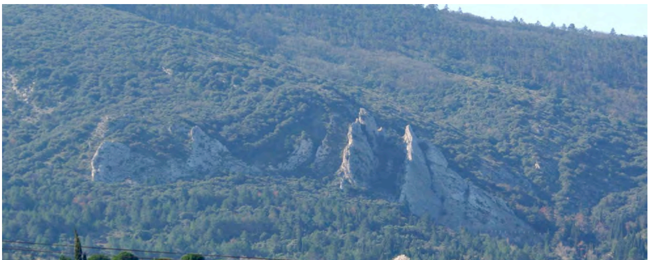
Pendages sub-verticaux sur le flanc nord de l'anticlinal de l'Alaric
