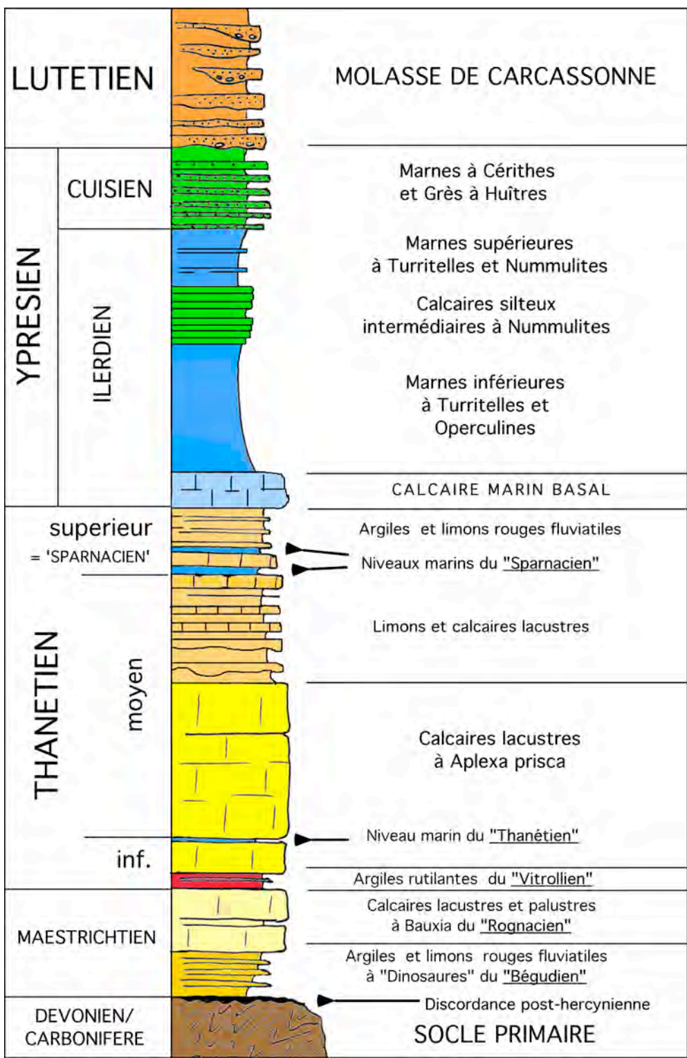
Log stratigraphique synthétique du Crétacé-Tertiaire de la Montagne d'Alaric
